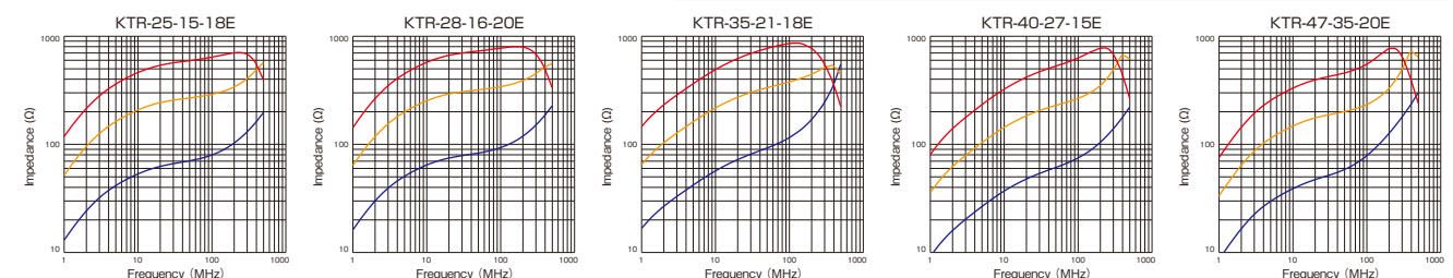
インピーダンス周波数特性 / Impedance vs frequency — 1ターン/Turn — 2ターン/Turn — 3ターン/Turn
