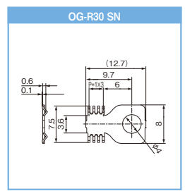
単位 / Unit: mm
